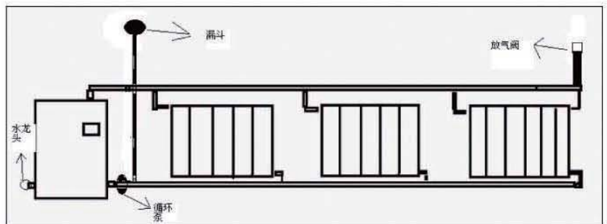
安装示意图
