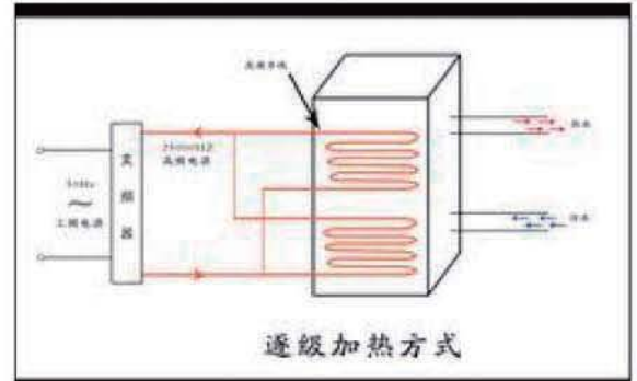
加热示意图
